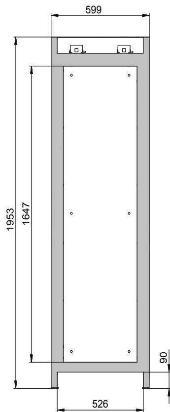
Frontalansicht
